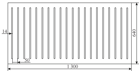
图3 受热面示意
