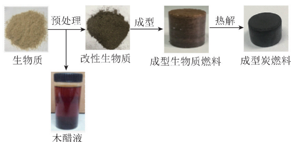
图3 生物质综合利用工艺路线2
