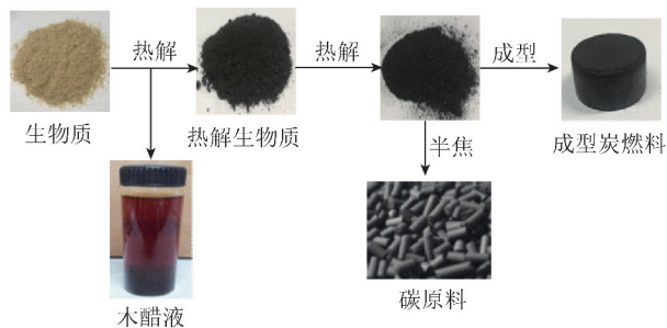
图2 生物质综合利用工艺路线1
