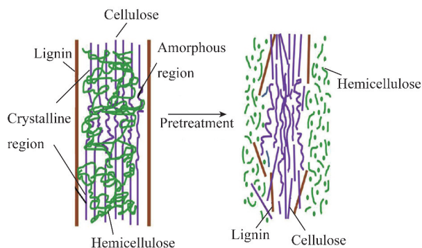
图1 预处理前后生物质细胞壁结构示意图 [10]
